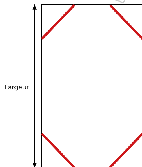
EN ANGLES : gabion de largeur 75 et 100 cm Distanceurs L445
