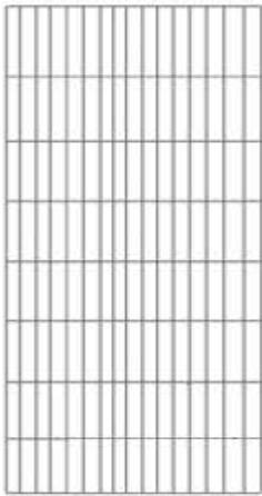
PANNEAU GRILLAGE • Maille 200 x 50 mm double fil • Crapal Premium
